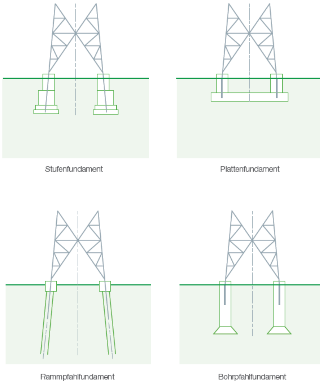
Abbildung 9 10: Schematische Darstellung von Gründungstypen
